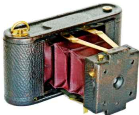
Folding Pocket Kodak, eerste model uit 1897. Rolfilmcamera voor 5,5 x 8 cm opnamen op daglichtspoel. Sluiter voor moment- en tijdopname, drie diafragma's op uittrekstrip, fixed focus lens.
